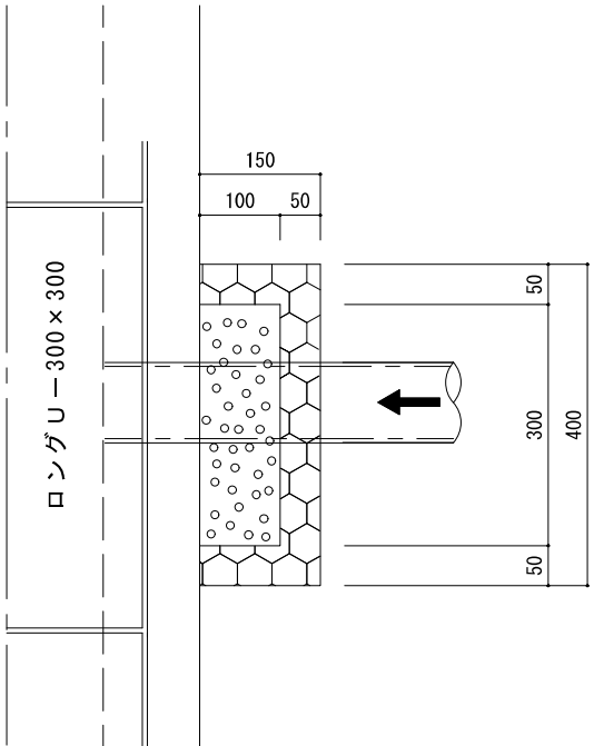
平面図
