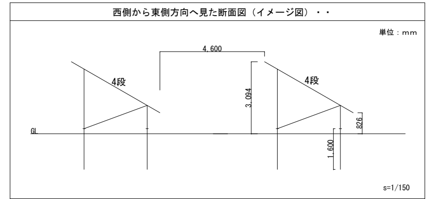
土地利用計画図 排水施設計画平面図、構造図 造成計画平面図、断面図
