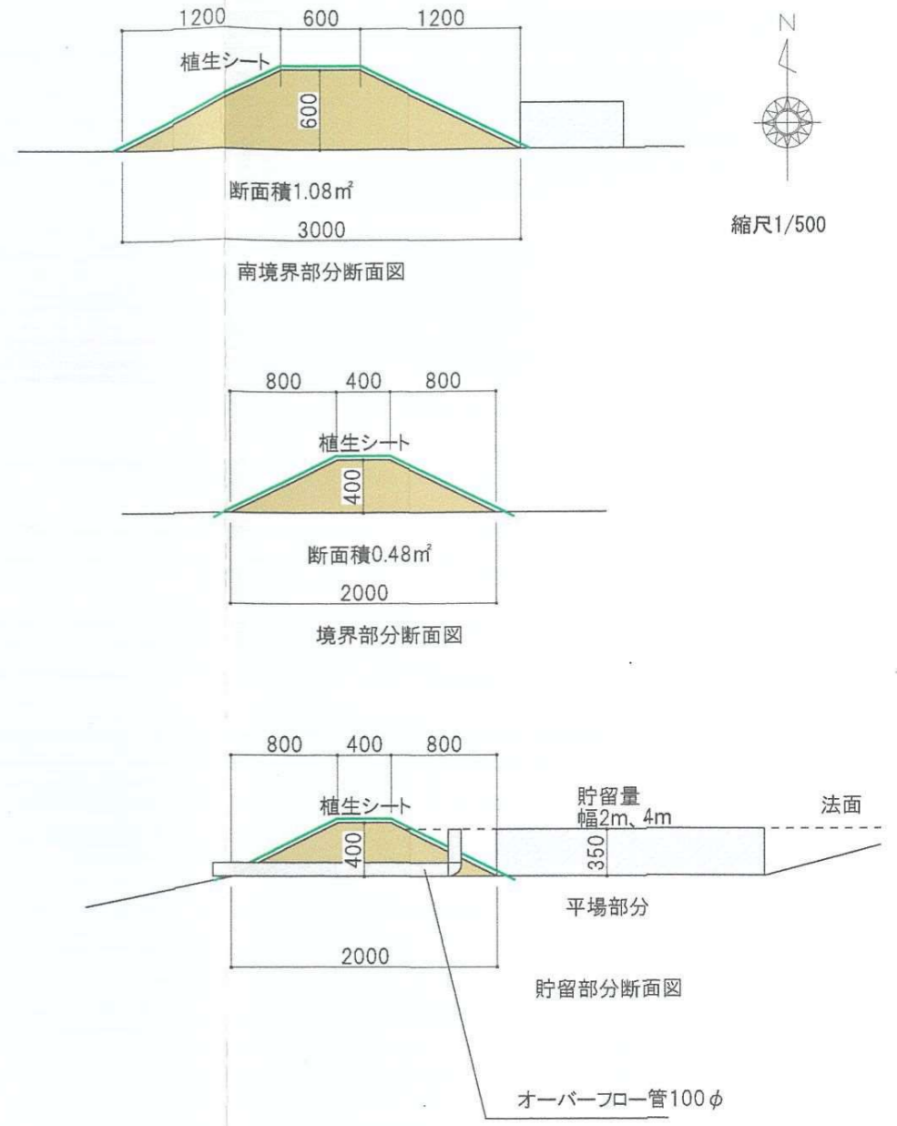
土地利用計画図 排水施設計画平面図、構造図 造成計画平面図、断面図
